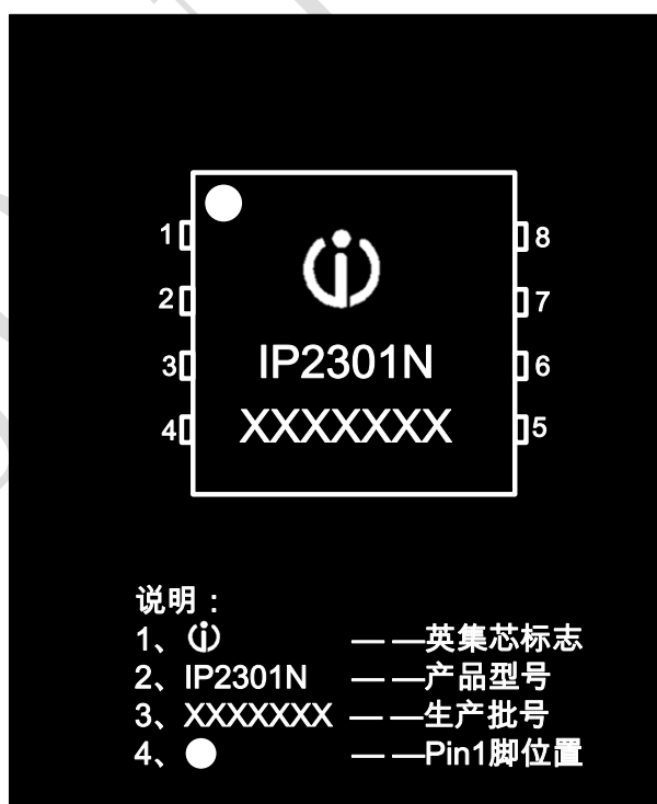
图 10 IP2301N IC 丝印说明(DFN8(0303))
