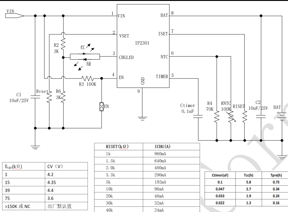
IP2301_DA2 双色灯应用原理图
