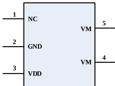
SOT23-5
