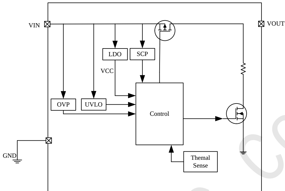
图 3 IP2615 内部系统框图
