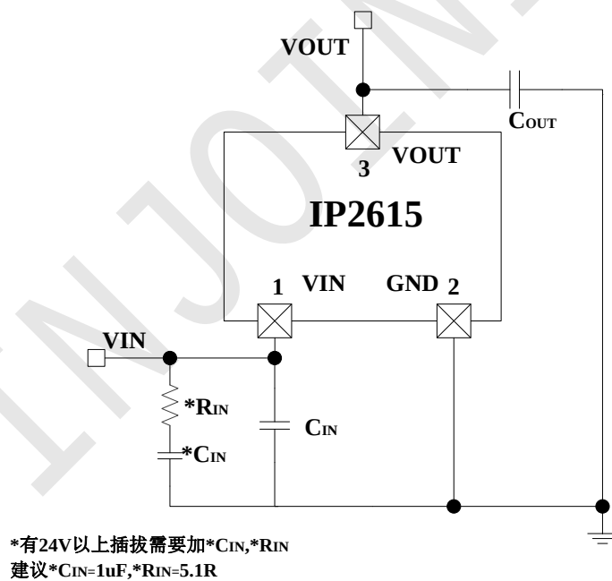
图 1 IP2615 简化应用原理图
