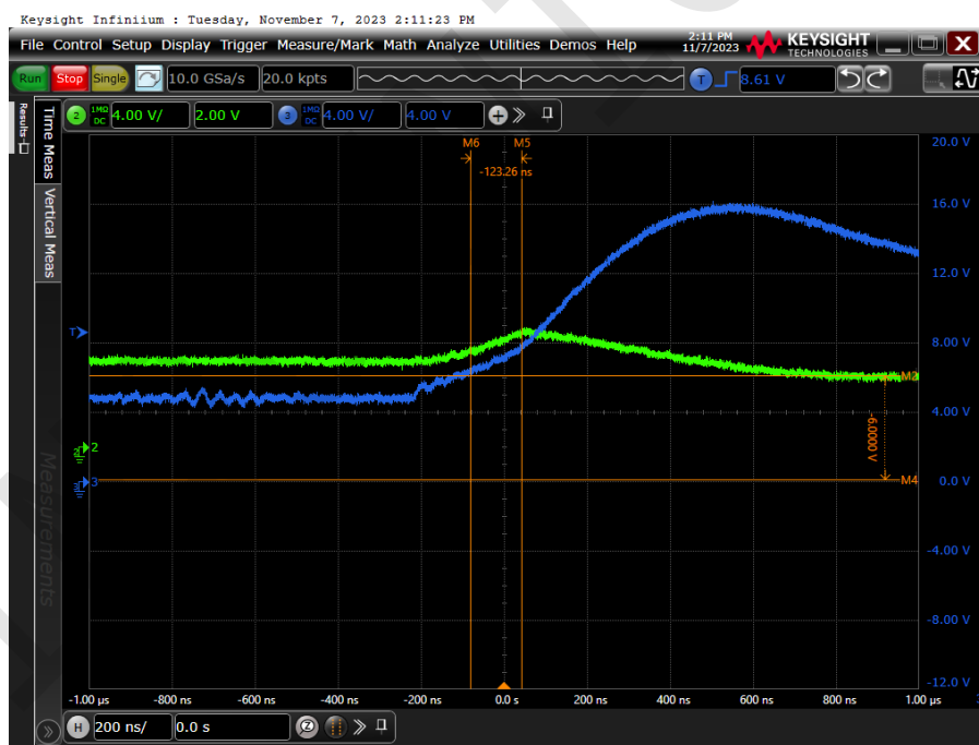
图 6 VIN 过压保护 (VIN=5V-15V)
