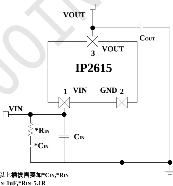
图 11 典型应用原理图
