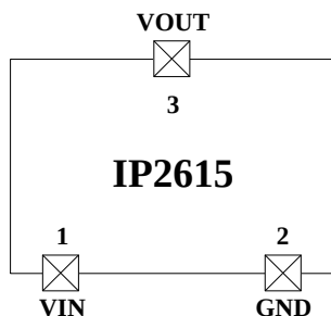
图 2 IP2615 引脚图
