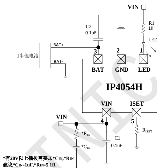
图 8 典型应用原理图
