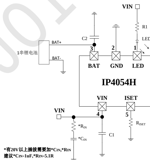
图 1 IP4054H 简化应用原理图
