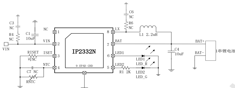
图 11 典型应用原理图
