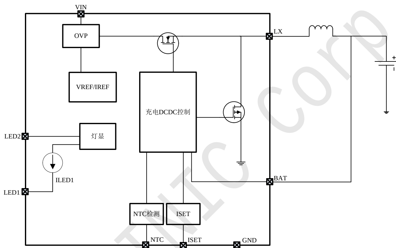
图 3 IP2332N 内部框图
