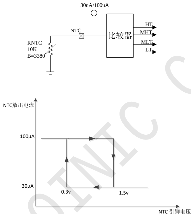
图 8 NTC 框图
