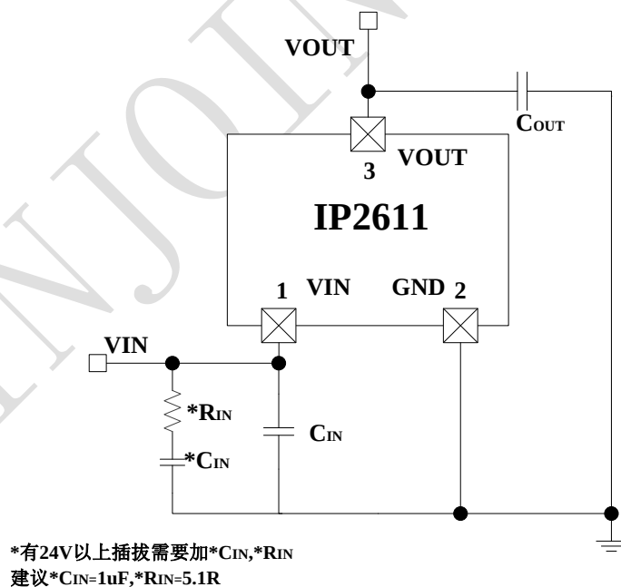
图 1 IP2611 简化应用原理图
