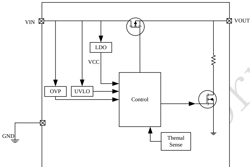
图 3 IP2611 内部系统框图
