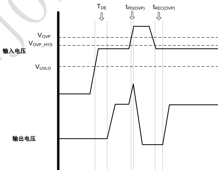
图 4 时序图
