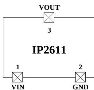
图 2 IP2611 引脚图
