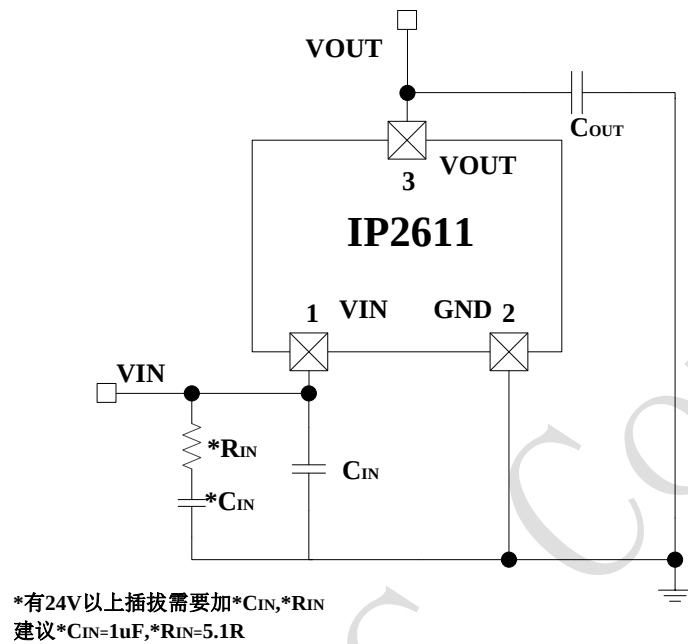
图 10 典型应用原理图
