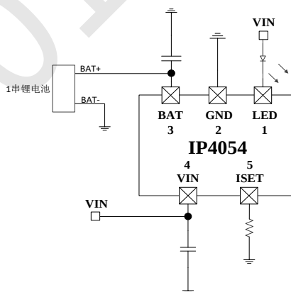
图 1 IP4054 简化应用原理图
