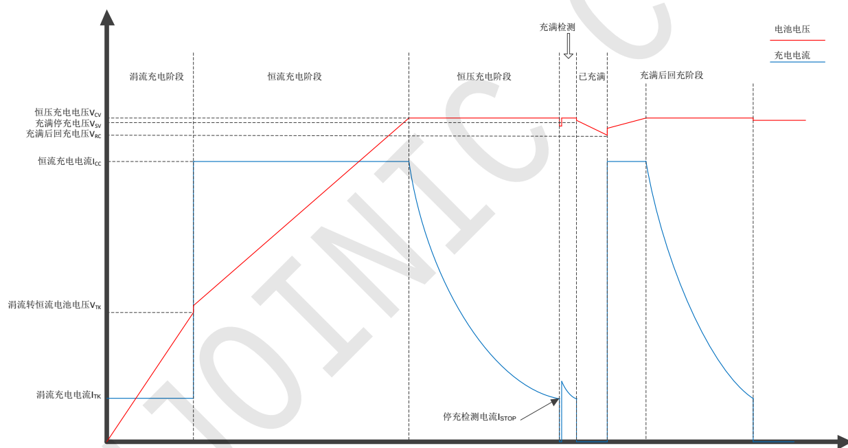
图 4 IP4054 充电过程示意图
