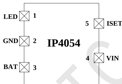
图 2 IP4054 引脚图
