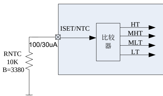
图 6 NTC 框图
