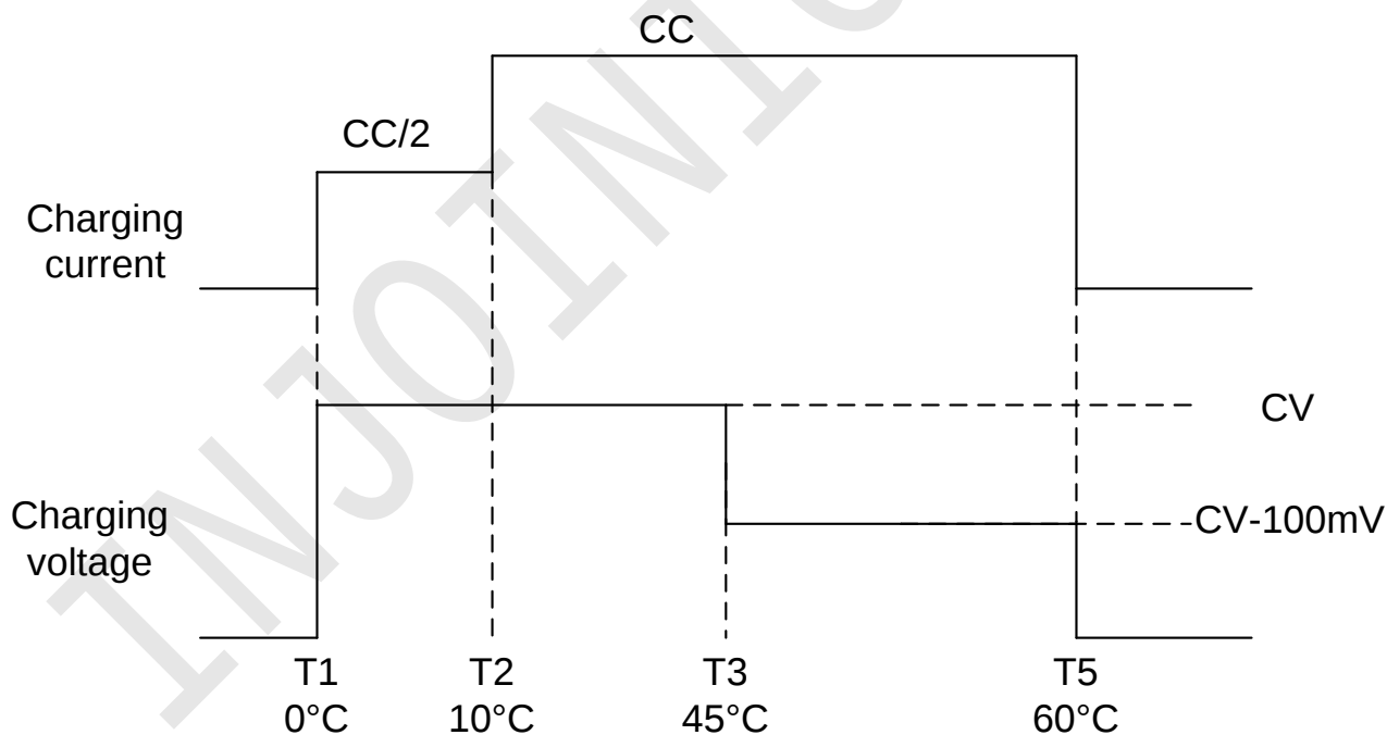
图 10 5 段式电池温度充电保护（兼容 JEITA 标准）示意图
