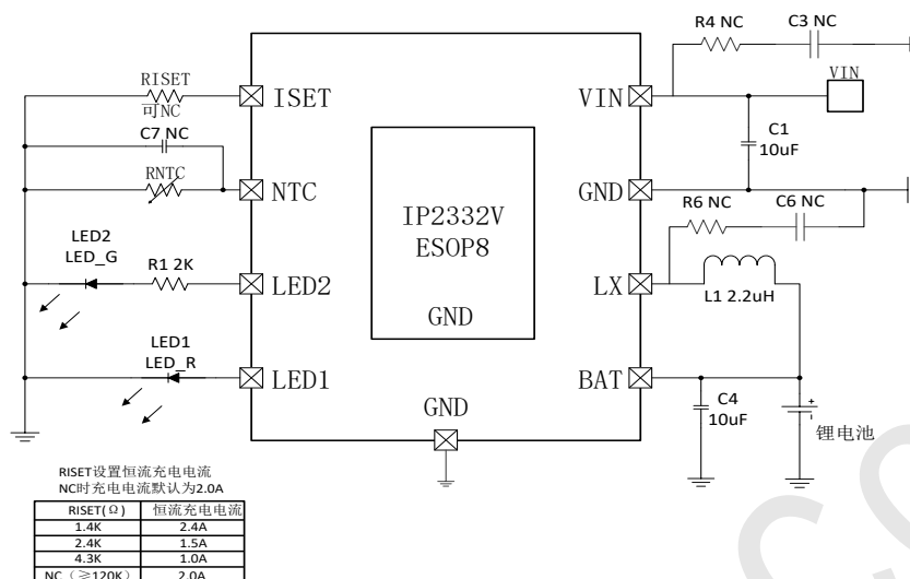
图 11 典型应用原理图
