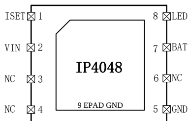
图 2 IP4048 引脚图
