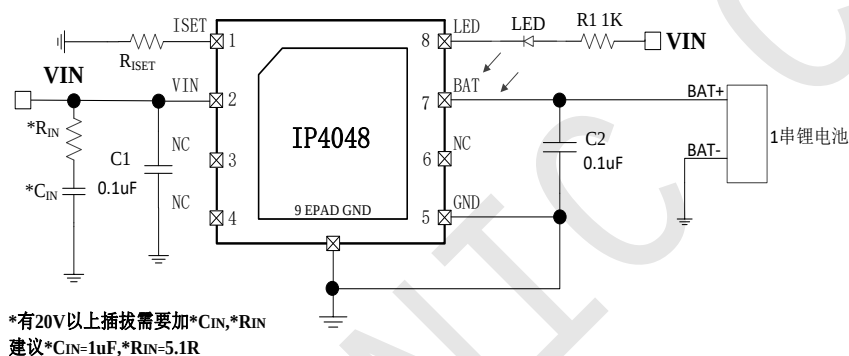
图 8 典型应用原理图
