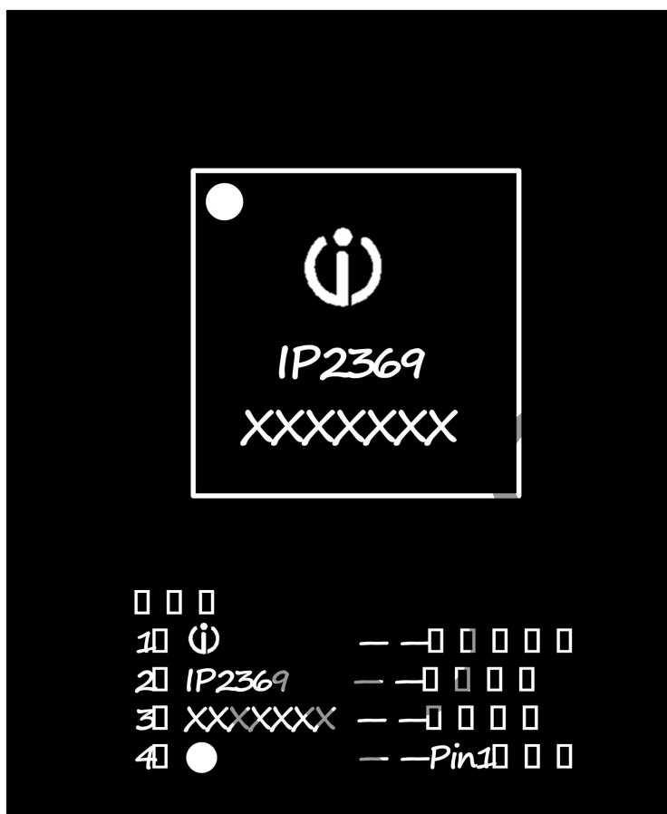
图 12 丝印图
